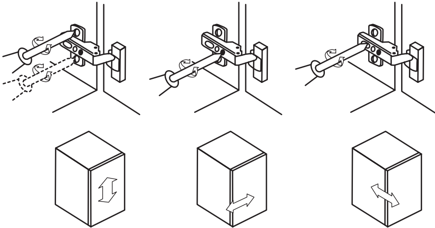
Регулировка дверок
