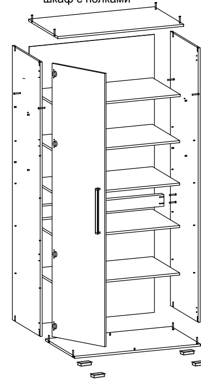
модель №8 (САИ 03.08) шкаф с полками
