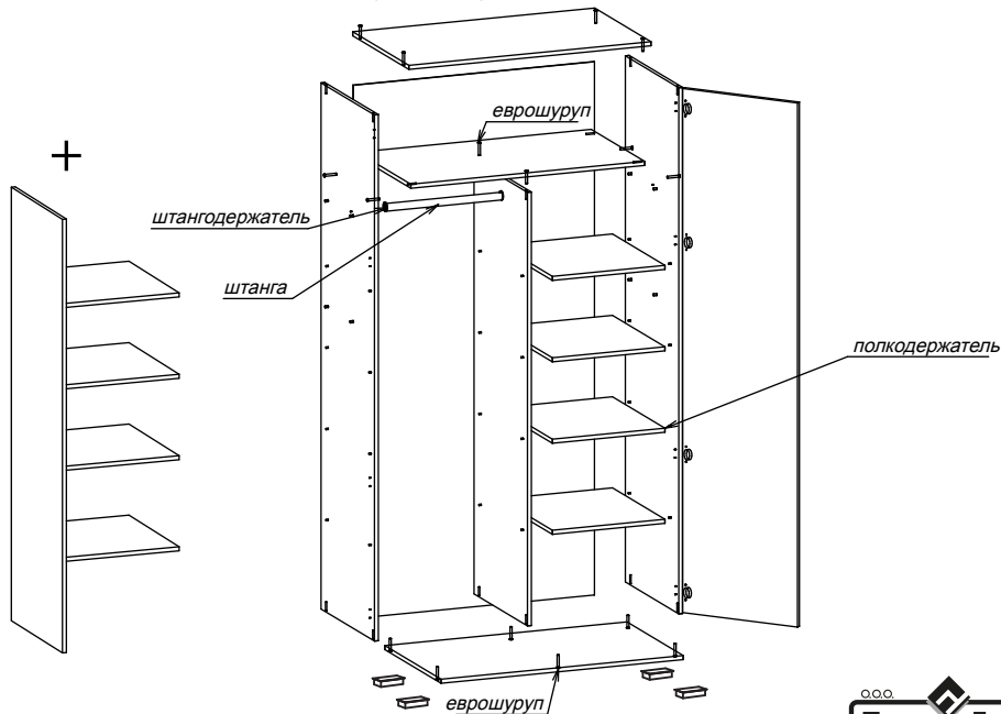
модель №9 (САИ 03.09) шкаф комбинированный
